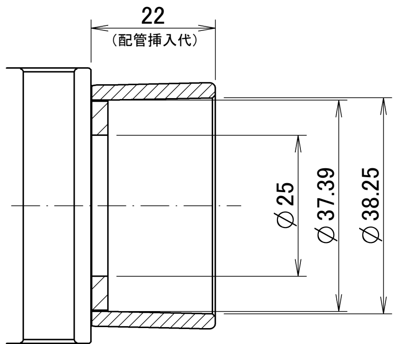
継手：受け口接合部寸法
