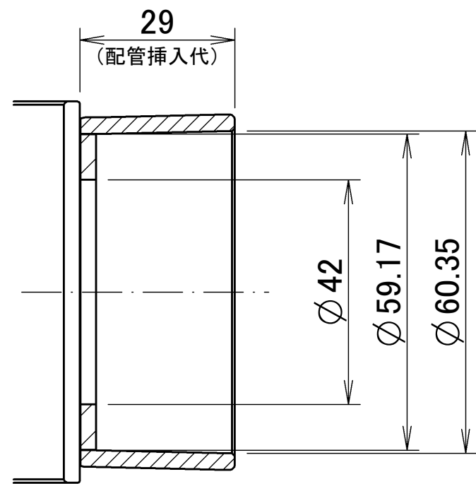
継手：受け口接合部寸法
