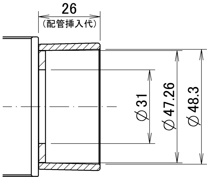
継手：受け口接合部寸法
