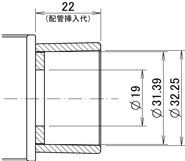
継手：受け口接合部寸法
