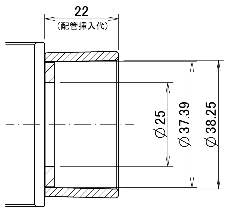
継手：受け口接合部寸法
