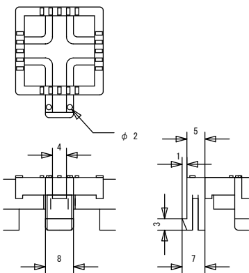
ジョイント オス (S=1/1)
