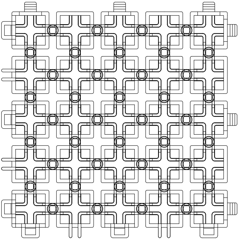
ジョイント オス (S=1/1)
