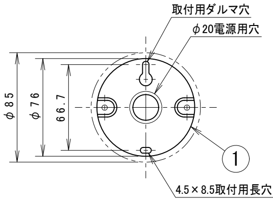
取付寸法(矢視a) (縮尺1/3)
