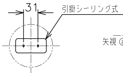
取付寸法 (矢視 (a))
