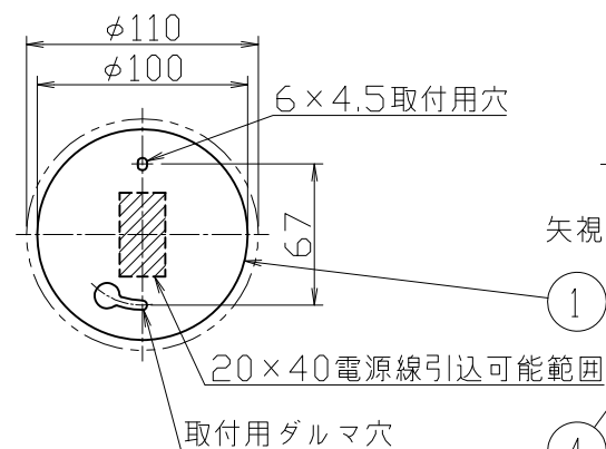
取付寸法（矢視 ㉑）
