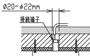
取付寸法(矢視 ②) (S=1/2)
