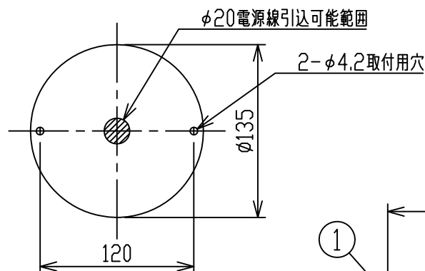
取付寸法(矢視 ②) (S=1/2)
