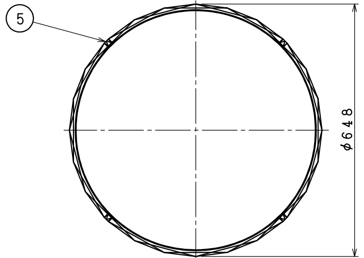
矢視(b)
