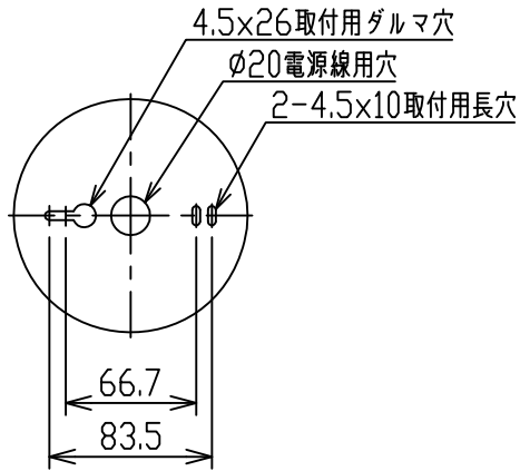
取付寸法(矢視①) S=1/2
