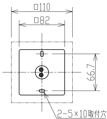
取付寸法(矢視a) (縮尺1/4)
