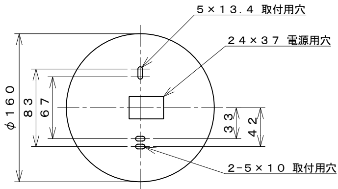
取付寸法 (矢視 a)
