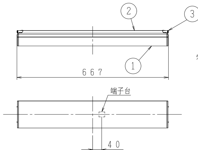
灯具最小施工寸法
