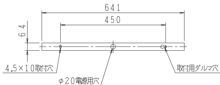
灯具最小施工寸法
