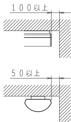
灯具最小施工寸法
