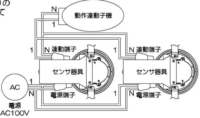
＜センサ器具2箇所検知+動作連動1台使用時の配線例＞
