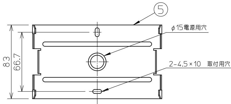
取付寸法 (矢視a)
