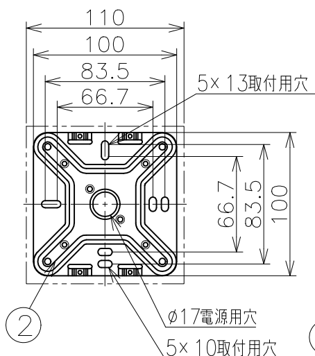
取付寸法 (矢視 ①)
