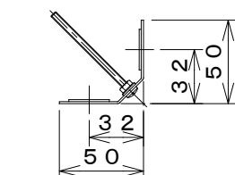
取付寸法 (矢視 a)
