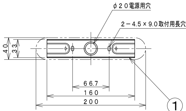
取付寸法 (矢視 a) (縮尺 1/4)
