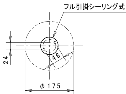
取付寸法(矢視a) (縮尺1/8)
