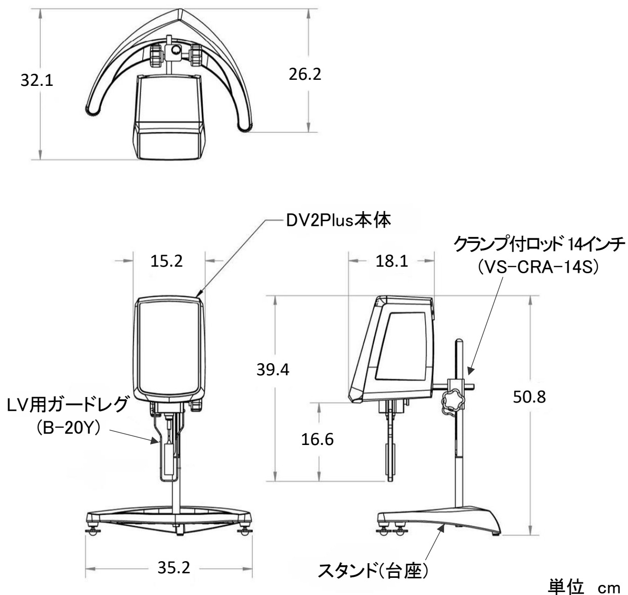
図面(外形寸法図)
