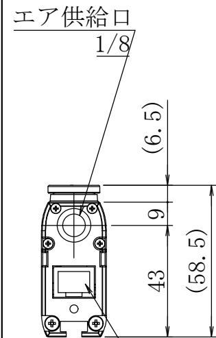
除電電極接続ケーブル用コネクタ
