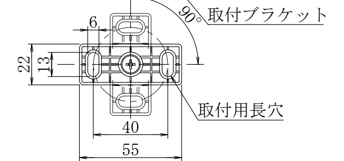
ブラケット取付時
