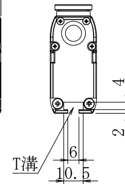
ブラケット取付時
