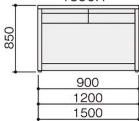
HTO-990H·1290H· 1590H
