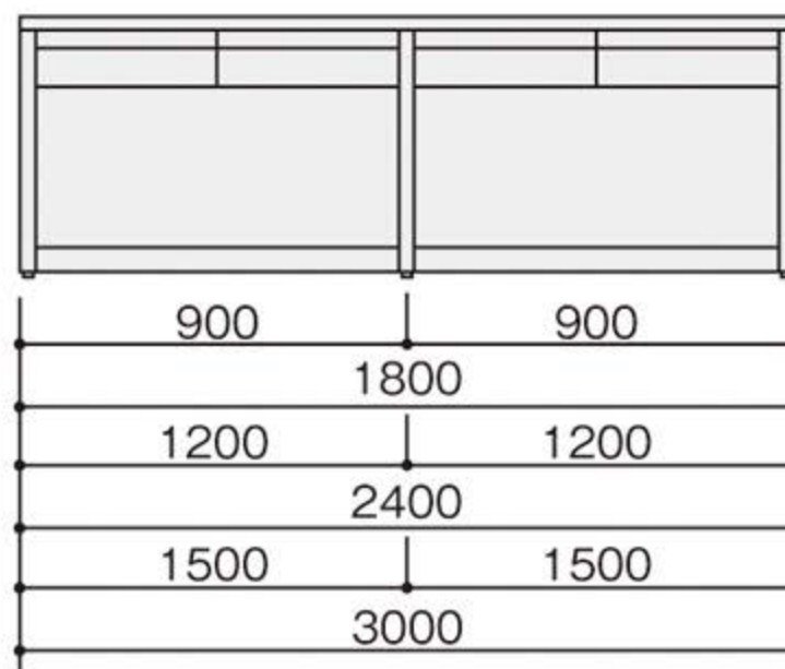
HTO-1890H·2490H·3090H
