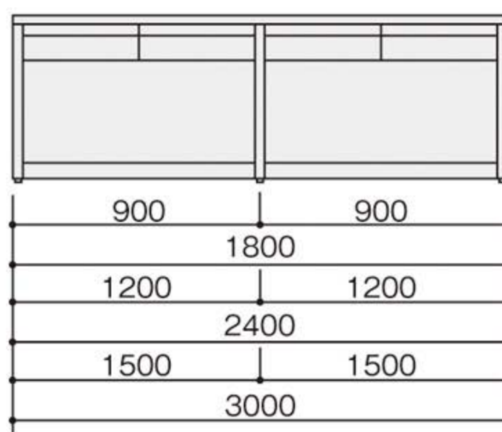
HTO-1860·2460·3060
