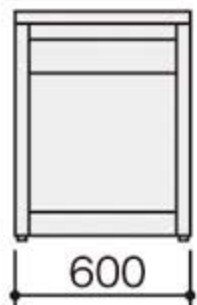
HTO-660
