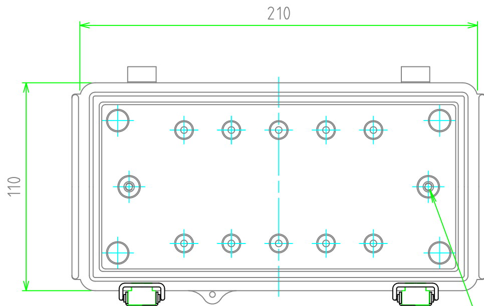
ボディ (内視) Base (Internal View)
