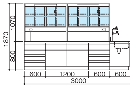
SBN-3012EG・3015EG
