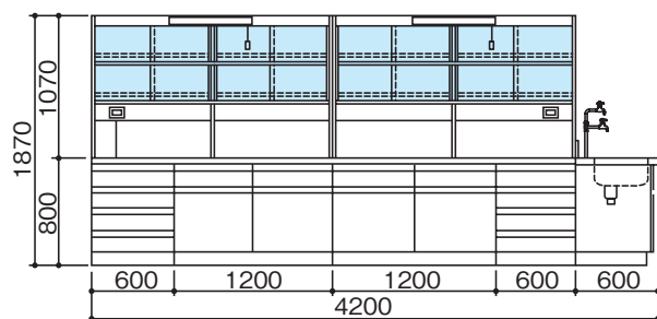
SBN-4212EG・4215EG
