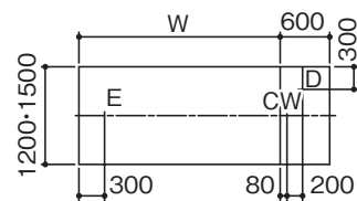
■配管・配線立上げ推奨位置図
