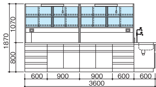
SBN-3612EG・3615EG
