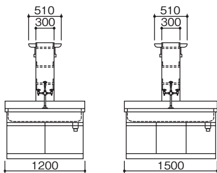
■配管・配線立上げ推奨位置図
