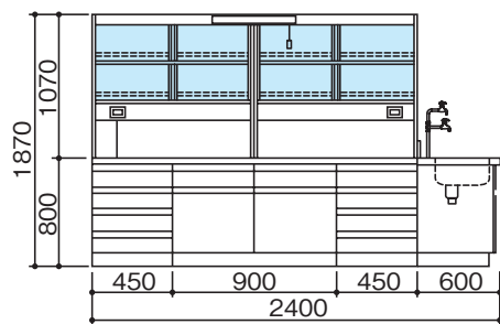
SBN-2412EG・2415EG
