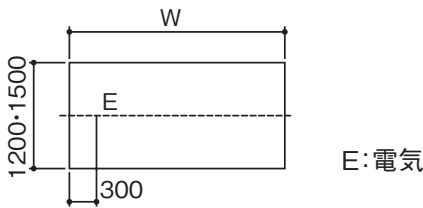
■配線立上げ推奨位置図
