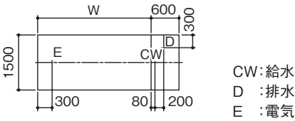
■配管・配線立上げ推奨位置図
