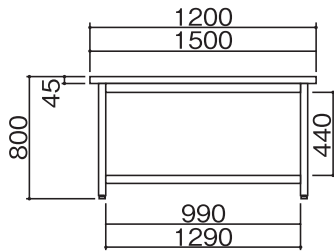
KSA-1275W · 1575W
