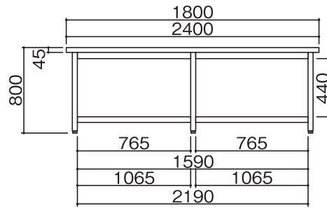
KSA-1875W · 2475W
