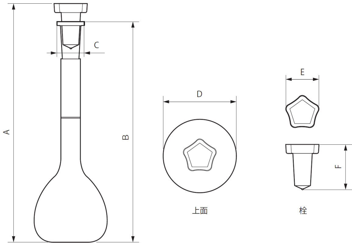
側面（栓装着）
