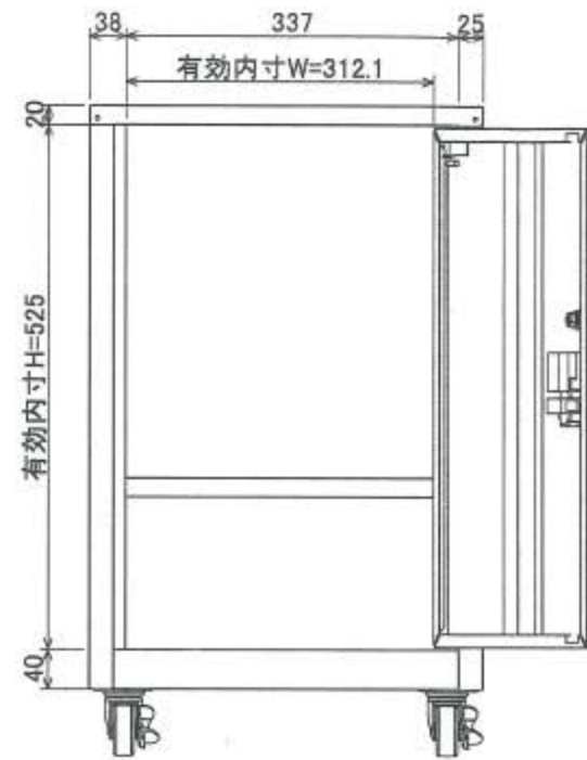
正面図(扉OPEN時)
