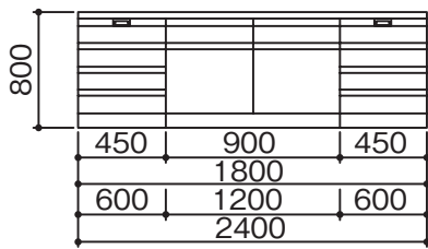
SQA-1875SD·2475SD
