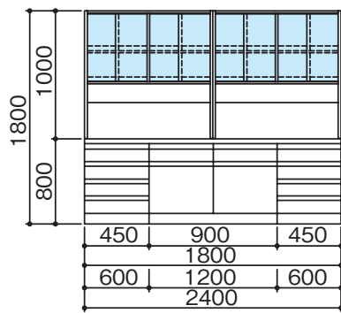
SQN-1875G·2475G
