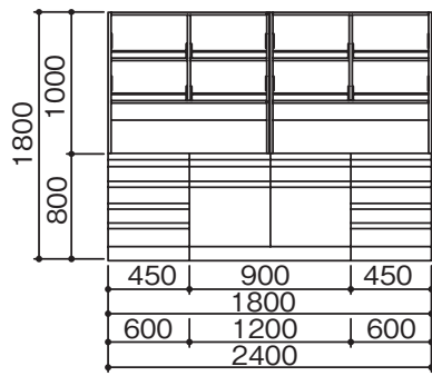
SQO-1875·2475
