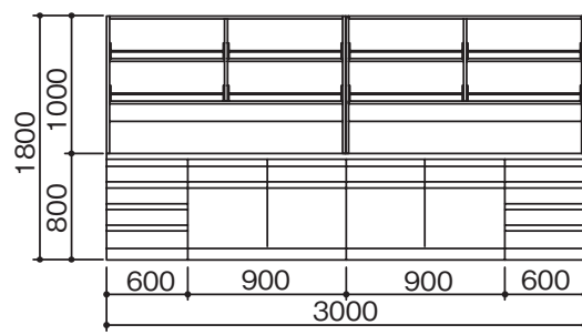
SQO-3075
