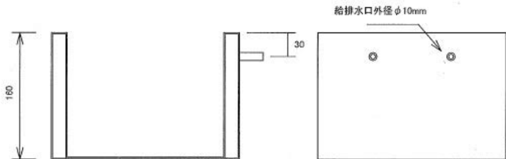
A-A断面
