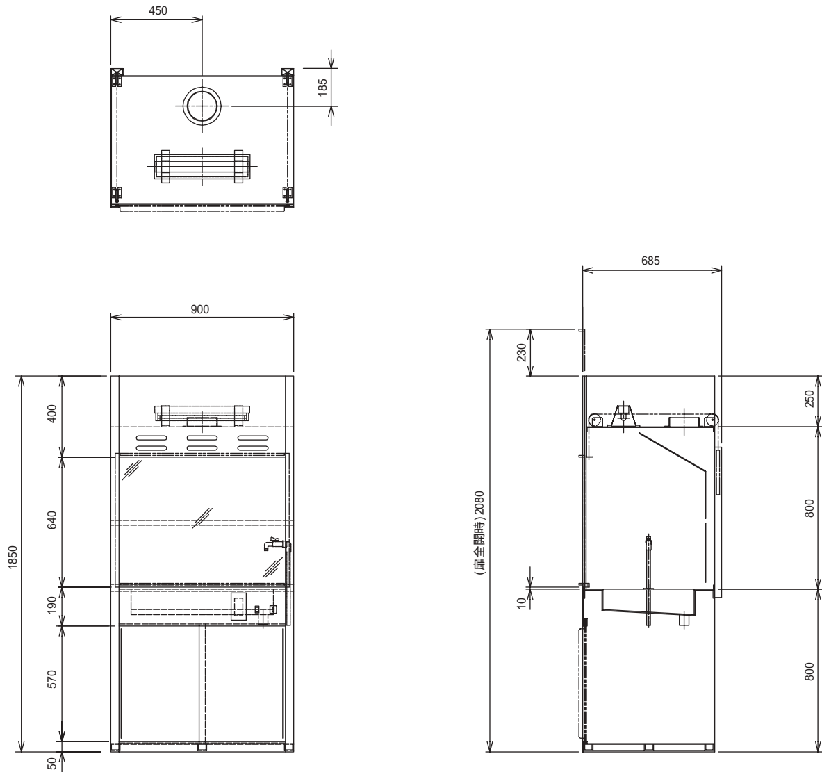
外形寸法図
