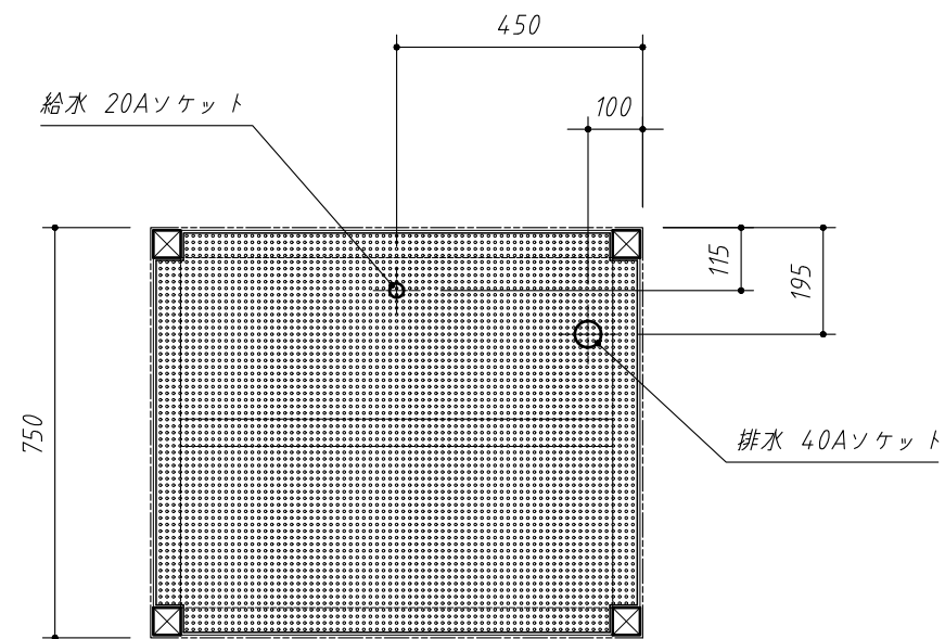
A断面図
