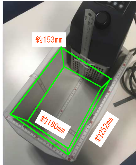
＜水槽設置時の有効内寸法＞
