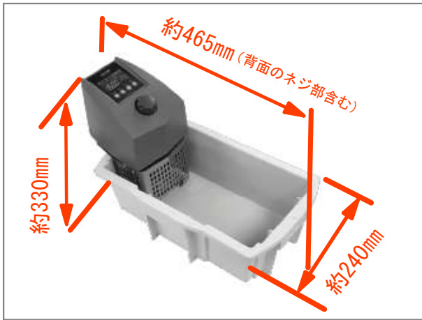
＜水槽設置時の外形寸法＞
