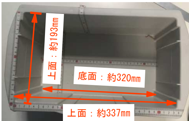
＜水槽のみ 有効内寸法＞
