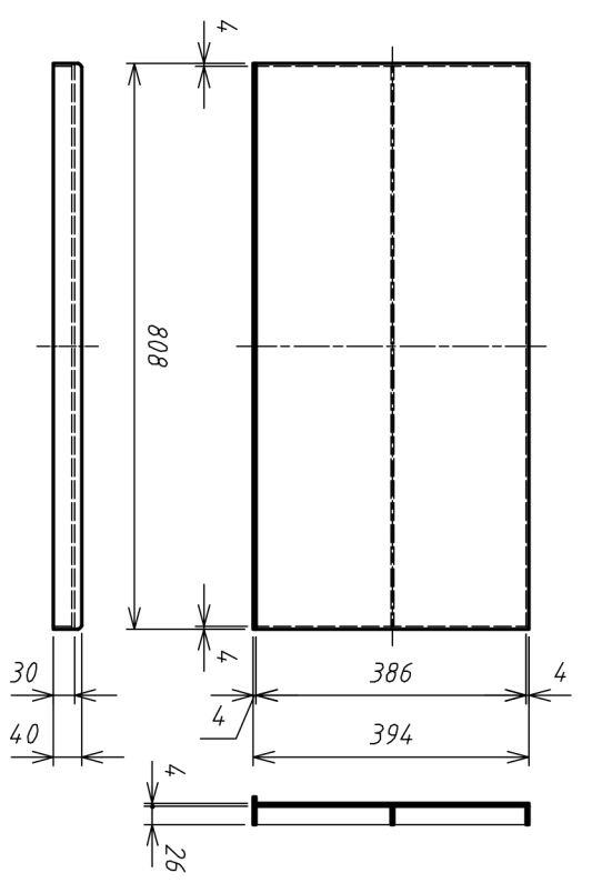
固定棚板寸法
