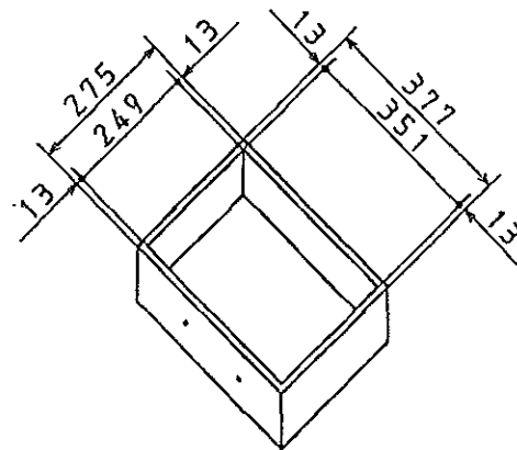
引出し寸法図
