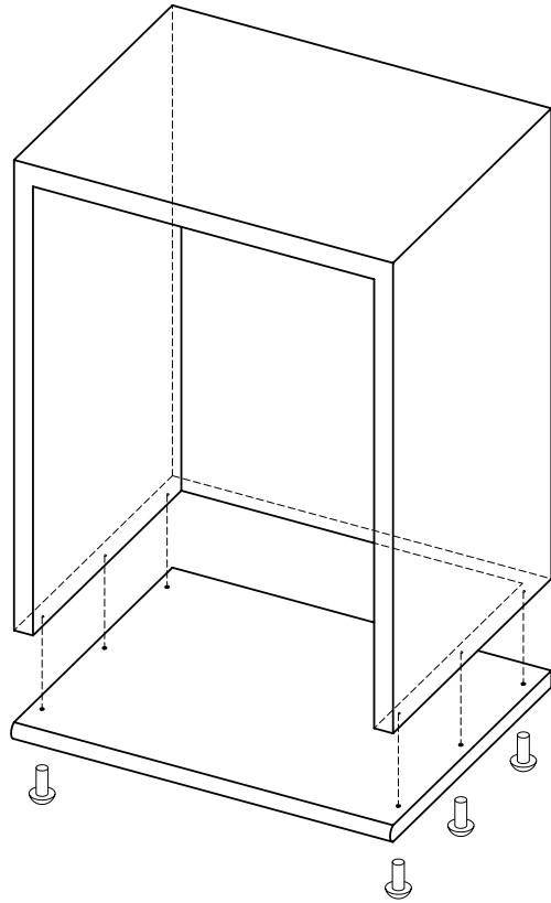
中段ユニット天板取付け図
