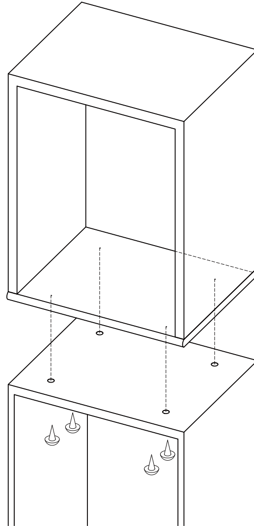
下段ユニット (D.475) 取付け図
