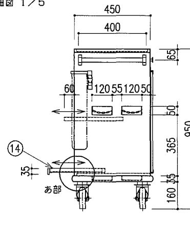
B 矢視図
