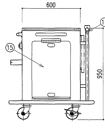
C 矢視図
