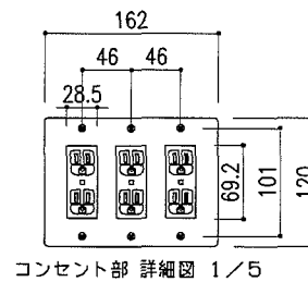
コンセント部 詳細図 1/5
